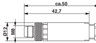
尺寸图
